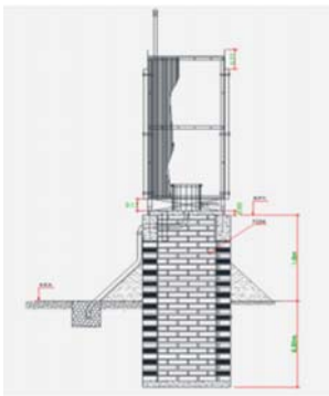
Letrina-semi elevada.
